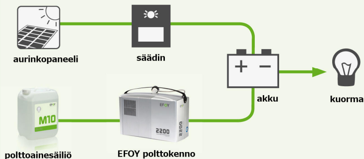
EFOY polttokenno + aurinkopaneeli + akku
